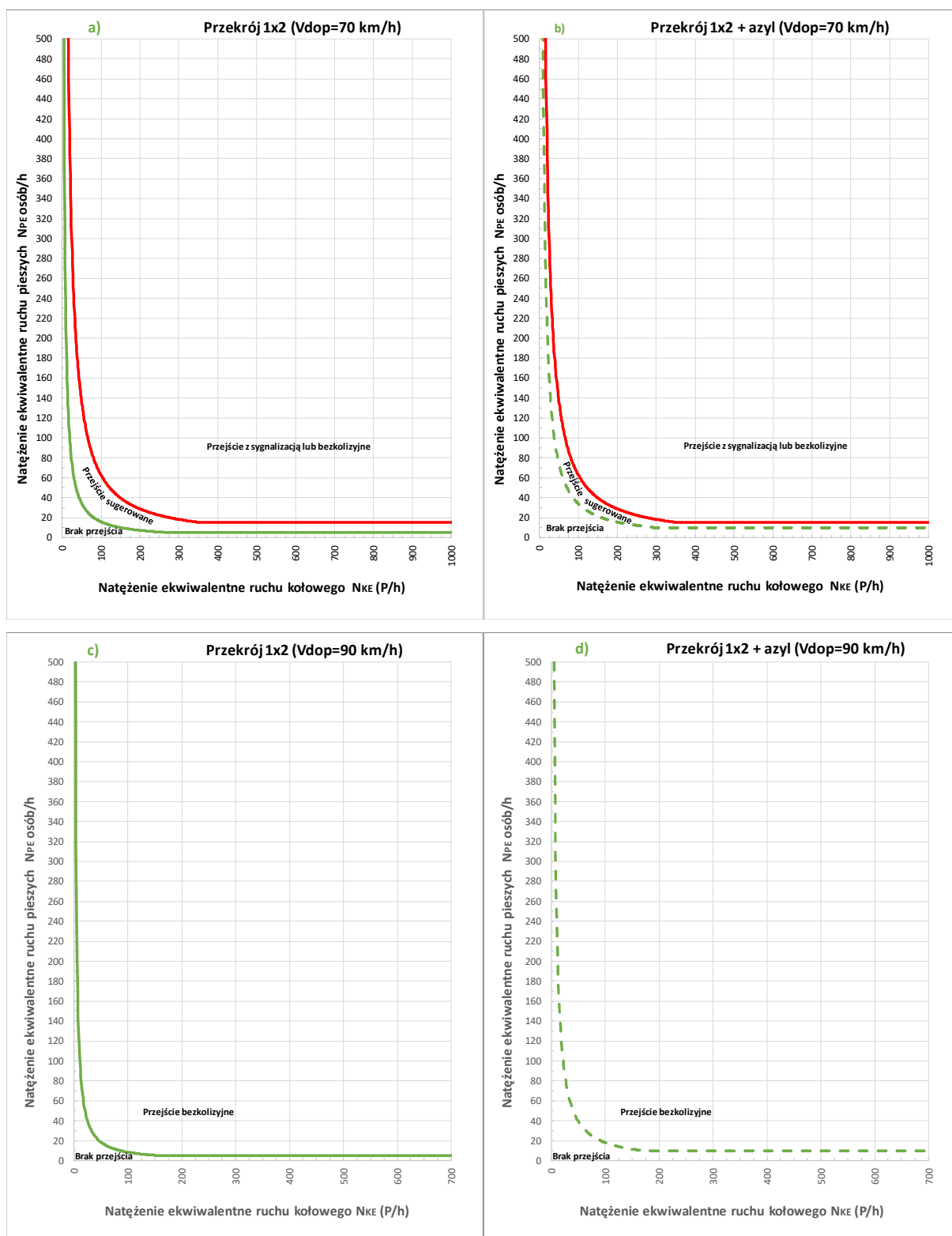
Rys. 8.4.2. Nomogram wyboru rodzaju infrastruktury punktowej dla pieszych przekraczających drogę o: a) V_{dop} = 70 \text{ km/h} bez wyspy azylu, b) V_{dop} = 70 \text{ km/h} z wyspą azylu, c) V_{dop} = 90 \text{ km/h} bez wyspy azylu, d) V_{dop} = 90 \text{ km/h} z wyspą azylu
