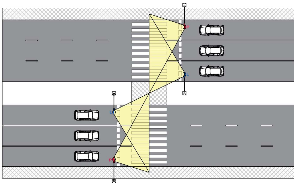
Rys. Z.3.8. Przykładowa lokalizacja opraw oświetleniowych na drodze dwujezdniowej o trzech pasach ruchu w jednym kierunku z pasem rozdzielającym (2/3) cztery oprawy, dwie oprawy z optyką lewą i dwie oprawy z optyką prawą
